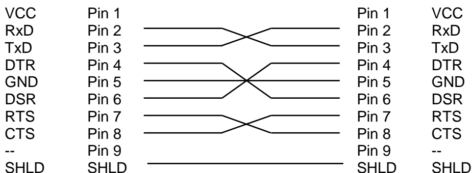
CR (DSUB9 female) (přes adaptér)
